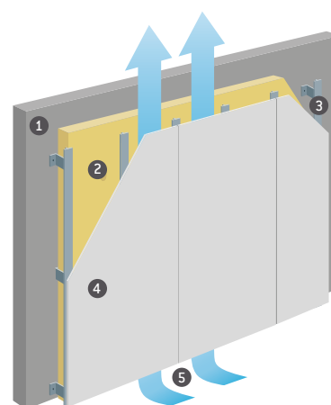
Principe de la façade rapportée ventilée
