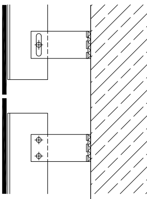
Variante 1: Profilstoß = Tafelfuge
