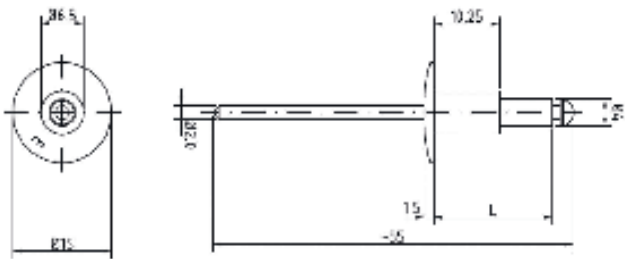
Алюминиевая заклепка
