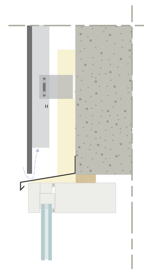
Figura 26: Connessione EQUITONE-Facciata Parte alta Parte bassa
