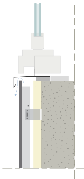
Figura 25: Connessione EQUITONE-Facciata continua continua
