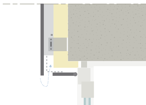
Figura 15: Chiusura superiore
