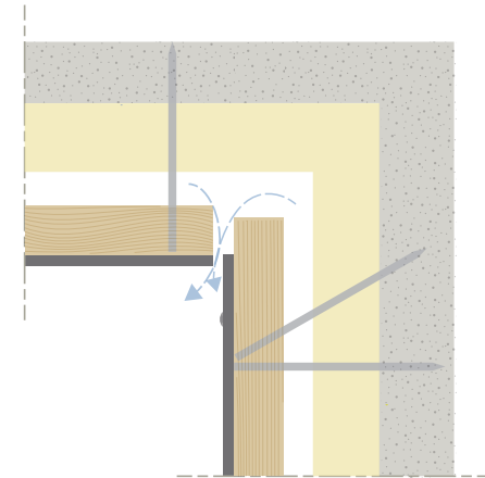
Figura 20: Dettagli soffitto
